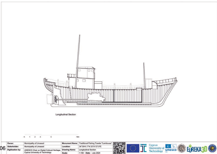
Figure 32. Longitudinal Section
