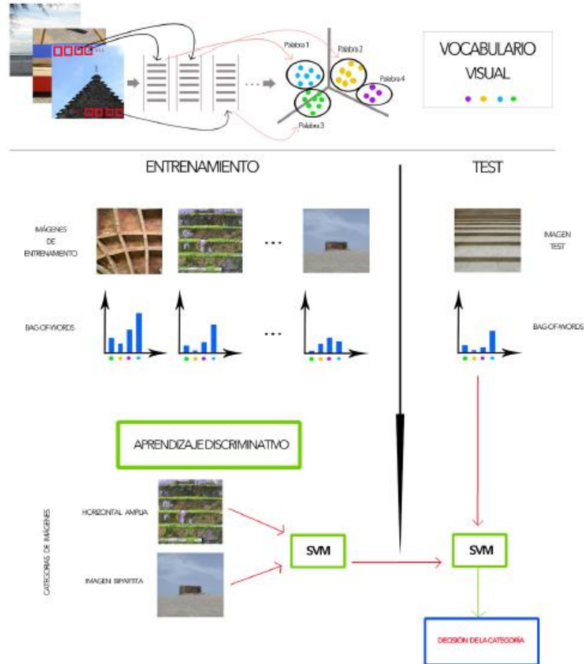
Figura 3.1. Esquema del programa de aprendizaje supervisado discriminativo.
